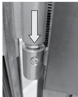
Při upevňování musí být vyfrézovaný povrch stavitelného válečku rovnoběžný s upínacím šroubem!
