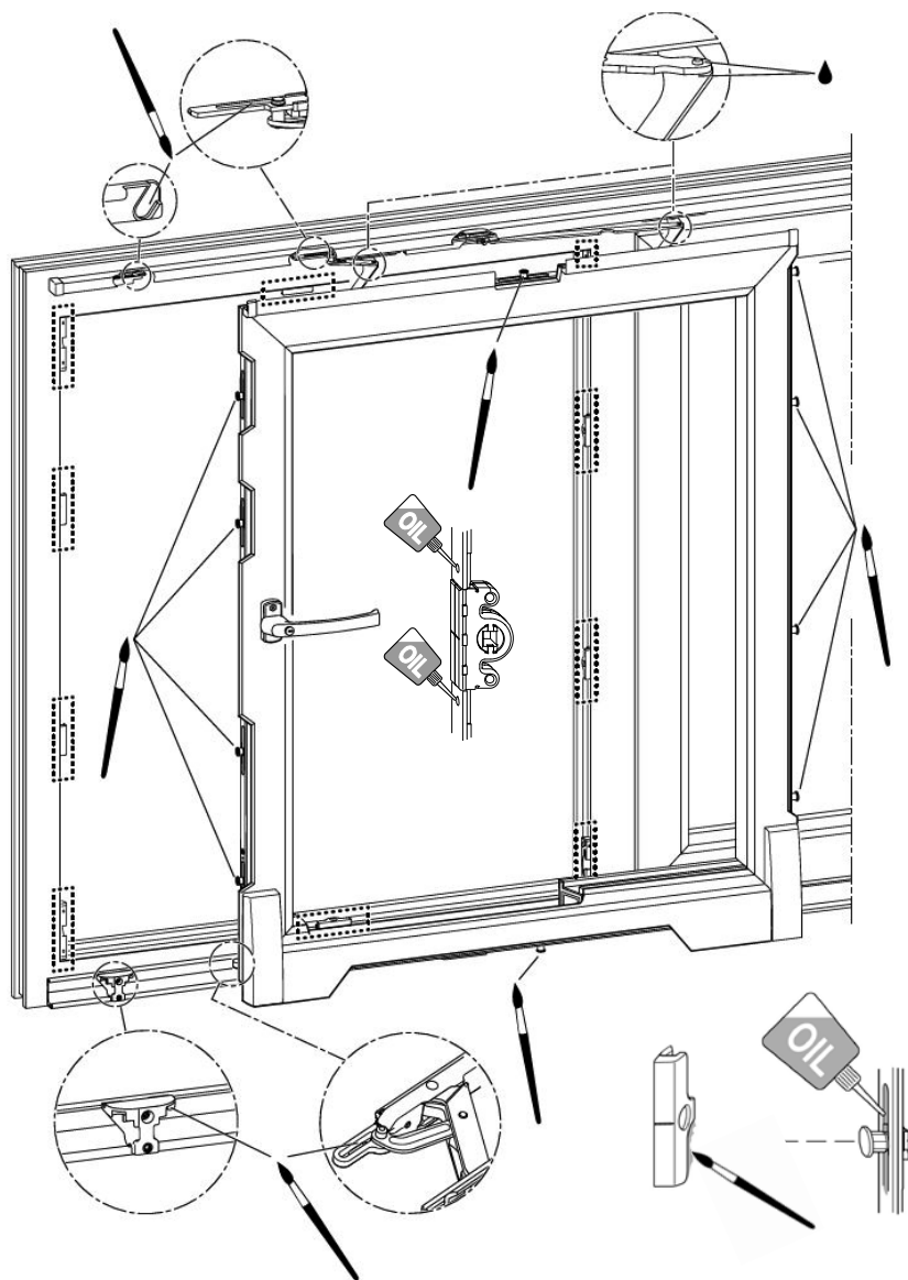
Mazací body na posuvných prvcích s odstavením:
