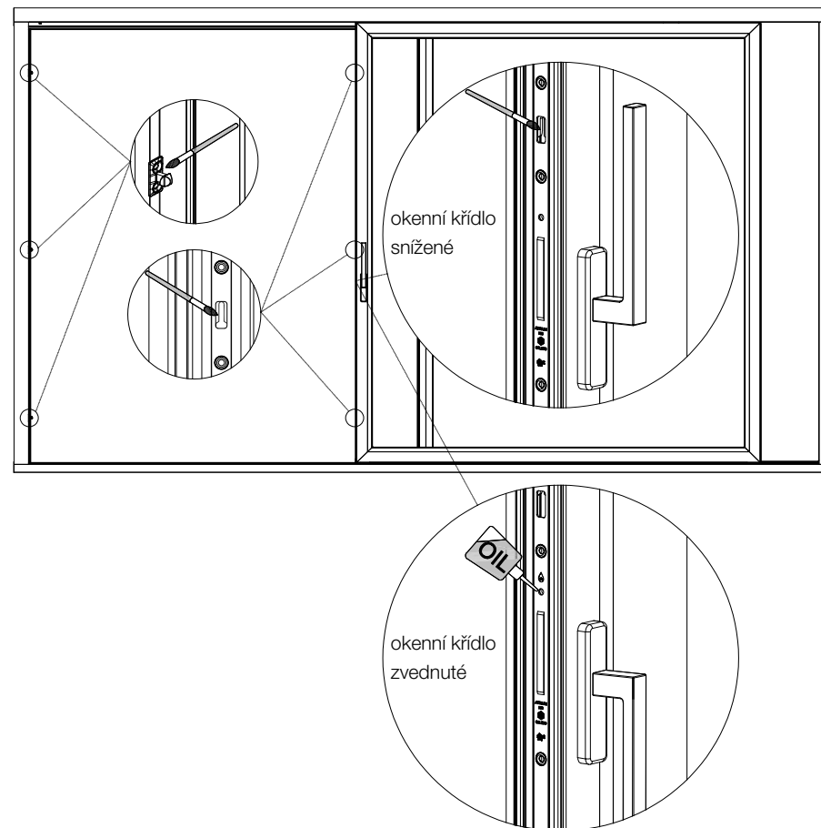
Mazací body na zdvižněposuvných dveřích:
